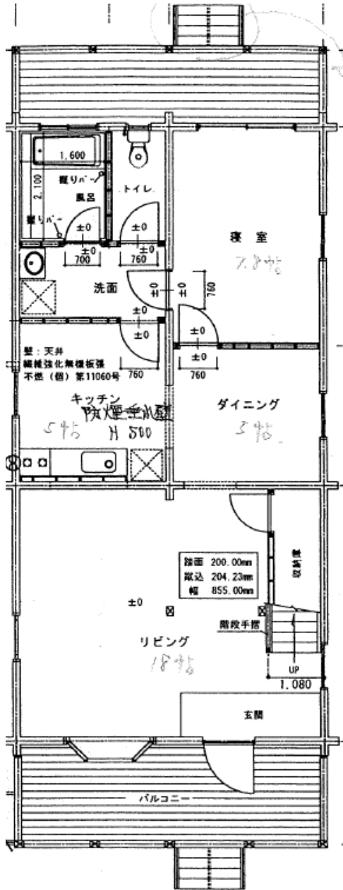
1階平面図
